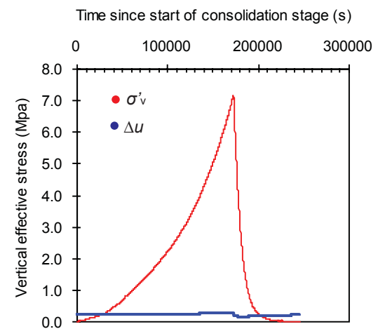
333-C0018A-17H-6, 20 cm
