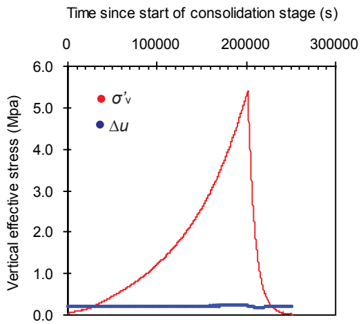
333-C0018A-7H-6, 0 cm
