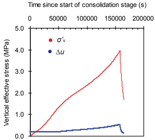
333-C0012C-10H-1, 105 cm
