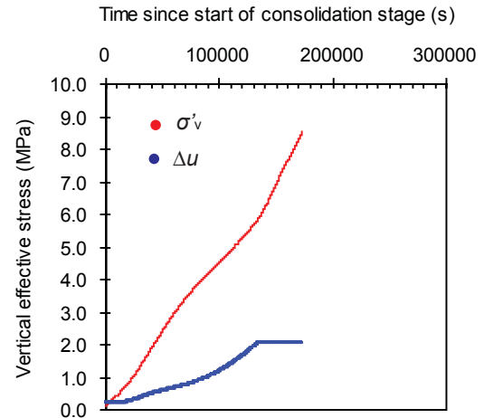
333-C0012D-10H-2, 89 cm
