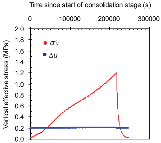
333-C0012C-6H-2, 60 cm
