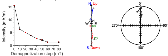
397-U1586A-17H-6, 49 cm | 156.83 m CSF-A | JR6 data
