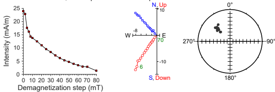
397-U1586A-16H-6, 74 cm | 147.72 m CSF-A | SRM data
