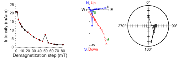
397-U1586A-27X-3, 28 cm | 208.52 m CSF-A | JR6 data
