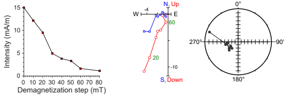
397-U1586A-29X-4, 77 cm | 223.32 m CSF-A | JR6 data
