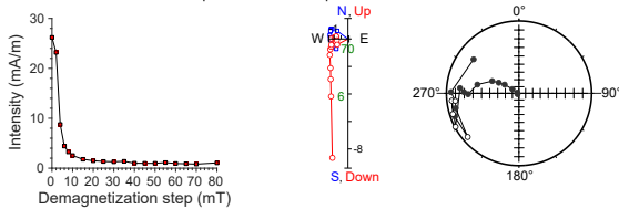
397-U1586A-28X-4, 69 cm | 216 m CSF-A | JR6 data
