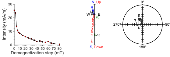
397-U1586A-20F-2, 63 cm | 179.53 m CSF-A | SRM data
