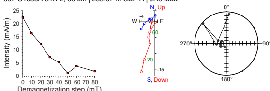
397-U1586A-31X-2, 38 cm | 239.37 m CSF-A | JR6 data
