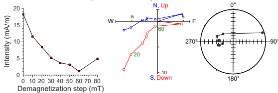
397-U1586A-30X-2, 33 cm | 229.62 m CSF-A | JR6 data
