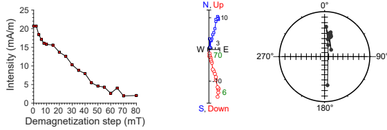
397-U1586A-36X-4, 103 cm | 291.48 m CSF-A | SRM data
