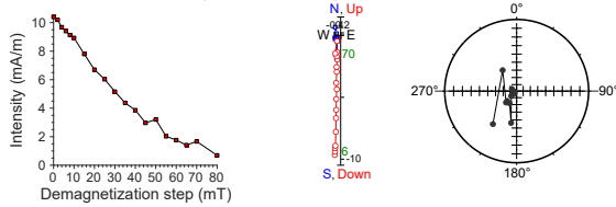
397-U1586A-36X-2, 74 cm | 288.24 m CSF-A | SRM data
