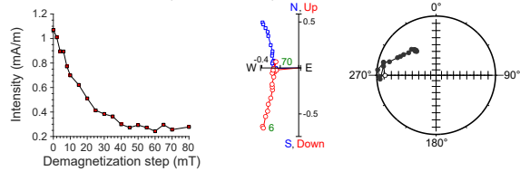
397-U1586A-37X-4, 99 cm | 301.21 m CSF-A | JR6 data
