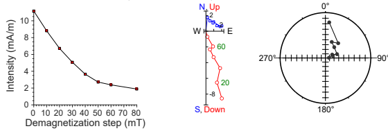
397-U1586A-37X-2, 18 cm | 297.39 m CSF-A | JR6 data
