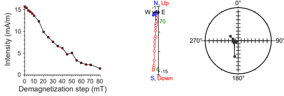
397-U1586A-34X-2, 57 cm | 268.68 m CSF-A | SRM data
