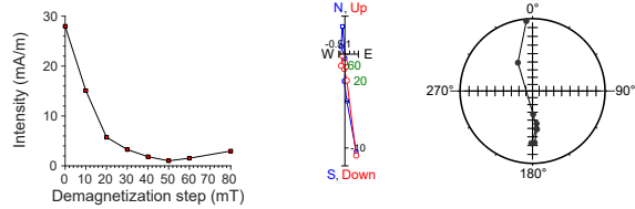
397-U1586A-37X-6, 28 cm | 303.5 m CSF-A | JR6 data
