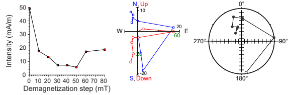
397-U1586A-38X-2, 26 cm | 307.17 m CSF-A | JR6 data
