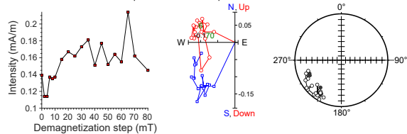
397-U1586A-38X-4, 51 cm | 310.44 m CSF-A | SRM data
