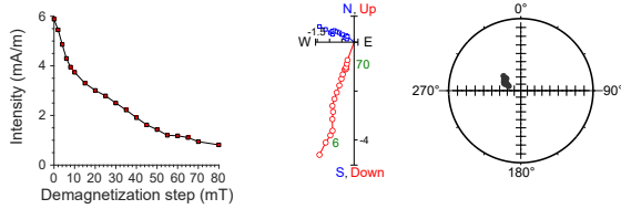
397-U1586A-36X-6, 81 cm | 294.16 m CSF-A | JR6 data
