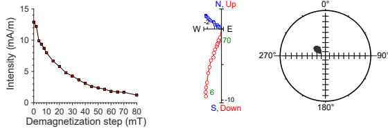
397-U1586A-33X-6, 64 cm | 265.03 m CSF-A | SRM data
