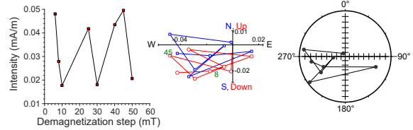
397-U1587B-21X-6, 77 cm | 192.16 m CSF-A | SRM data
