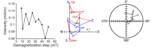
397-U1587B-15X-3, 74 cm | 137.13 m CSF-A | JR6 data
