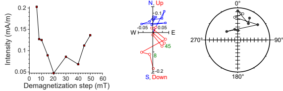
397-U1587B-16X-4, 74 cm | 148.33 m CSF-A | JR6 data
