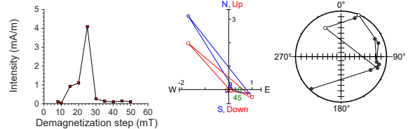
397-U1587B-20X-2, 75 cm | 184.16 m CSF-A | SRM data
