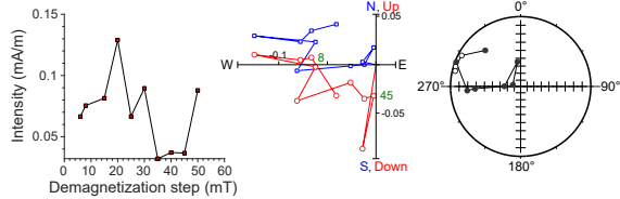
397-U1587B-18X-4, 90.5 cm | 167.905 m CSF-A | SRM data
