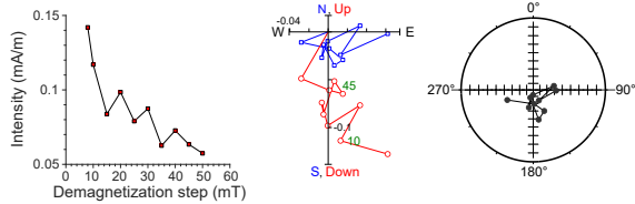
397-U1587B-14X-3, 74 cm | 127.49 m CSF-A | SRM data
