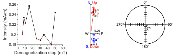
397-U1587B-19X-3, 61 cm | 175.8 m CSF-A | SRM data
