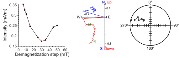
397-U1587B-14X-2, 74 cm | 125.99 m CSF-A | SRM data
