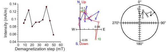
397-U1587B-14X-4, 74 cm | 129 m CSF-A | SRM data
