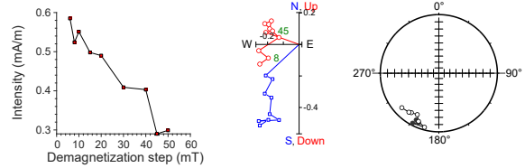
397-U1587B-14X-4, 24 cm | 128.5 m CSF-A | SRM data
