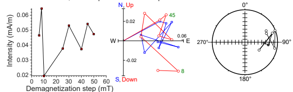
397-U1587B-21X-6, 108 cm | 192.47 m CSF-A | SRM data
