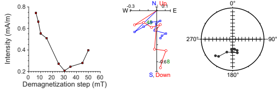
397-U1587B-14X-2, 129 cm | 126.54 m CSF-A | SRM data
