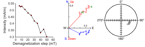
397-U1587B-25X-4, 82 cm | 221.32 m CSF-A | SRM data
