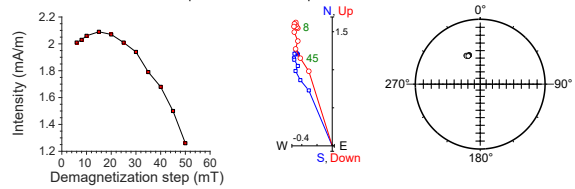
397-U1587B-26X-4, 103 cm | 231.23 m CSF-A | SRM data
