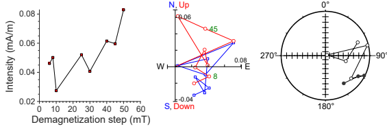
397-U1587B-21X-7, 42 cm | 193.21 m CSF-A | SRM data
