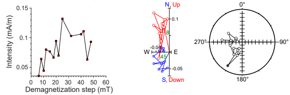
397-U1587B-28X-3, 95 cm | 249.06 m CSF-A | SRM data
