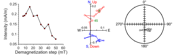
397-U1587B-24X-2, 95 cm | 215.46 m CSF-A | SRM data
