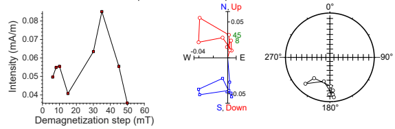
397-U1587B-27X-2, 74 cm | 237.65 m CSF-A | SRM data
