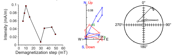
397-U1587B-27X-2, 47.5 cm | 237.385 m CSF-A | SRM data
