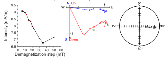
397-U1587B-59X-3, 50 cm | 541.6 m CSF-A | SRM data
