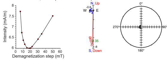
397-U1587B-57X-5, 33 cm | 524.9 m CSF-A | SRM data
