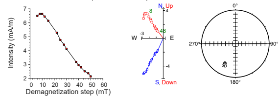
397-U1587B-59X-5, 58 cm | 544.67 m CSF-A | SRM data
