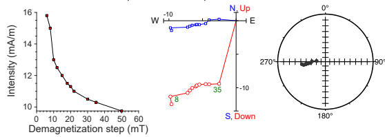
397-U1587B-57X-6, 84 cm | 526.91 m CSF-A | SRM data
