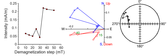
397-U1385G-21X-3, 63 cm | 187.54 m CSF-A | JR6 data
