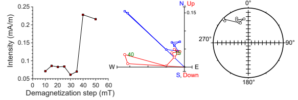
397-U1385G-20X-5, 137 cm | 181.6 m CSF-A | JR6 data
