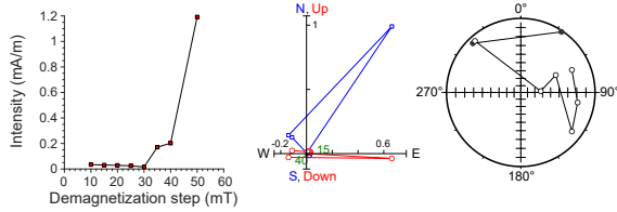
397-U1385G-20X-4, 71 cm | 179.44 m CSF-A | JR6 data
