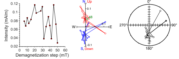
397-U1385G-28X-3, 90 cm | 255.7 m CSF-A | SRM data
