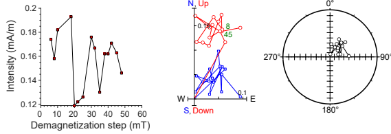
397-U1385G-24X-5, 52 cm | 218.4 m CSF-A | SRM data
