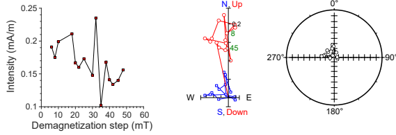
397-U1385G-19X-4, 74 cm | 169.75 m CSF-A | JR6 data
