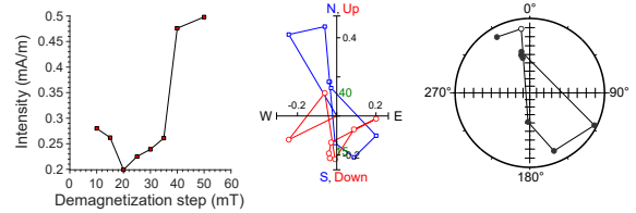
397-U1385G-22X-4, 81 cm | 198.93 m CSF-A | JR6 data
