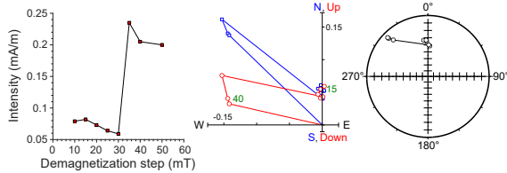
397-U1385G-23X-4, 59 cm | 208.42 m CSF-A | SRM data
