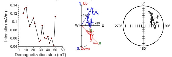
397-U1385G-30X-4, 42 cm | 276.15 m CSF-A | JR6 data
