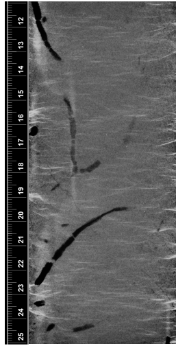
U1385G-10H-3, 18 cm
