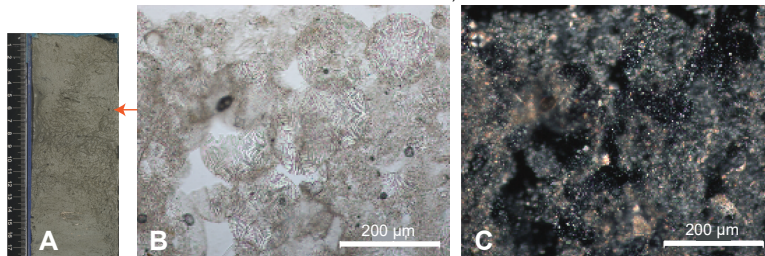
U1588C-20X-2, 94-113 cm
